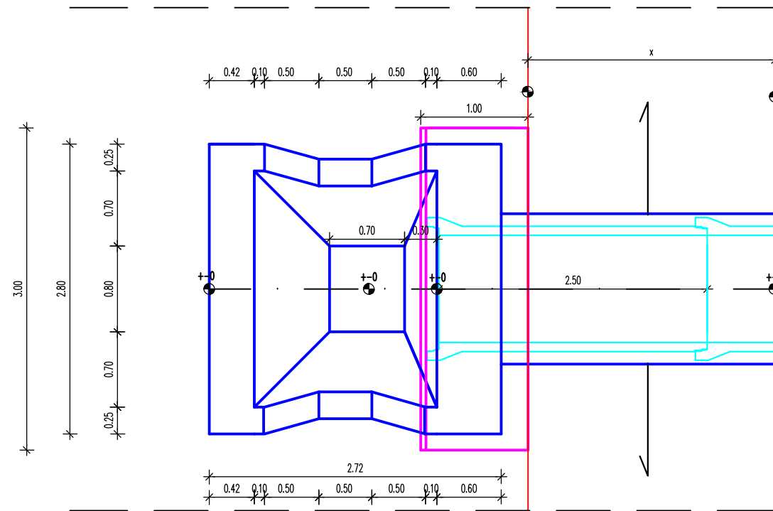
M=1:50 ОСНОВА ВЛЕЗНО КАЗАНЧЕ
