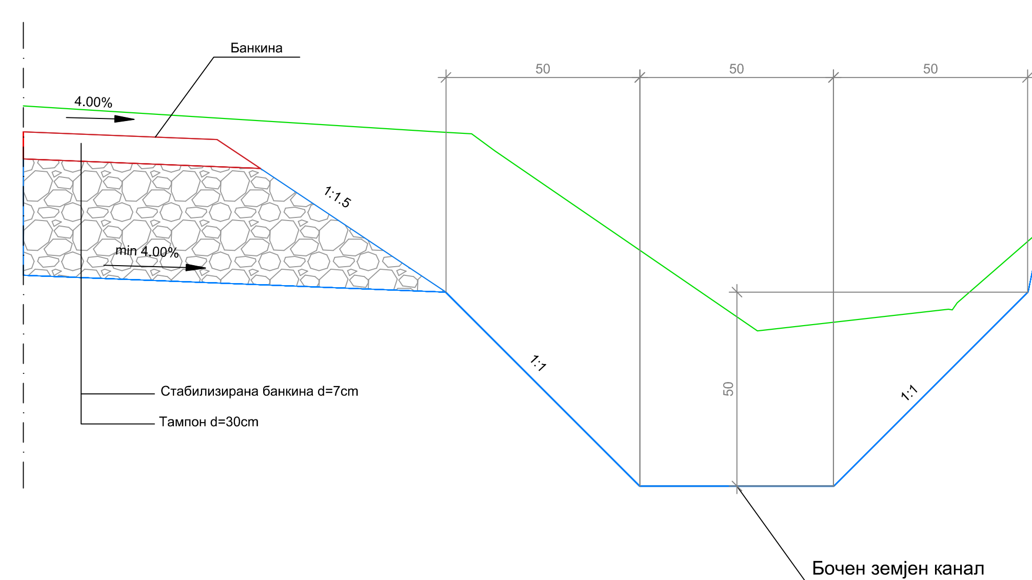
Деталъ "С" R = 1:10
