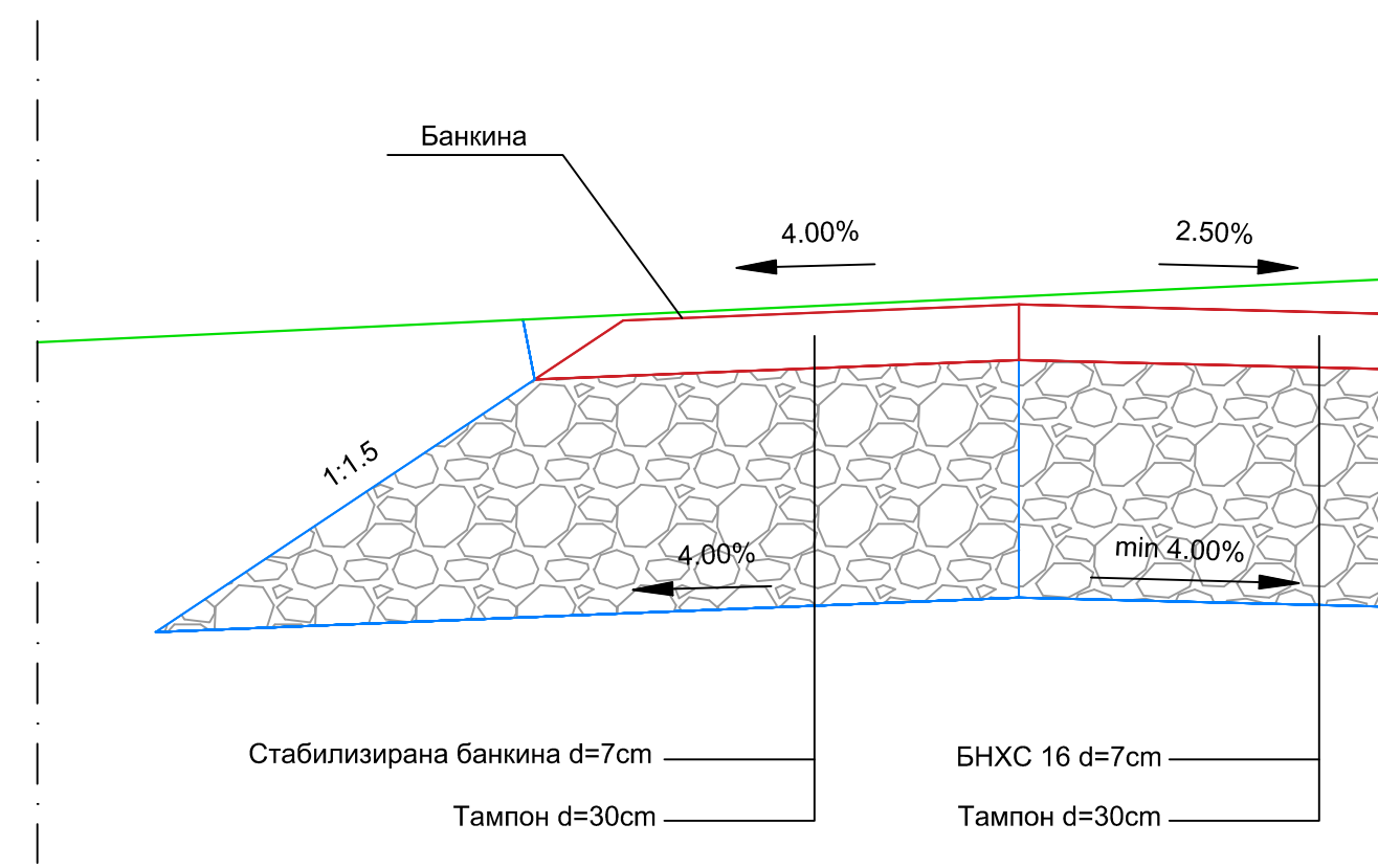
Деталъ "А1" R = 1:10
