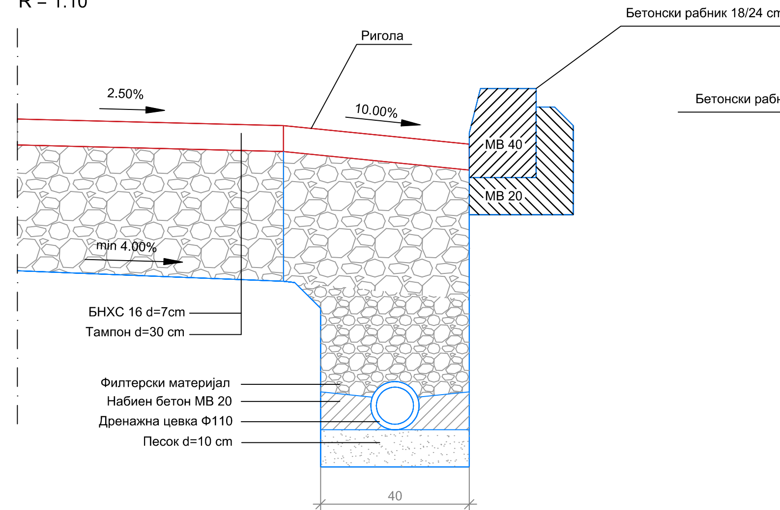
Деталъ "D" R = 1:10
