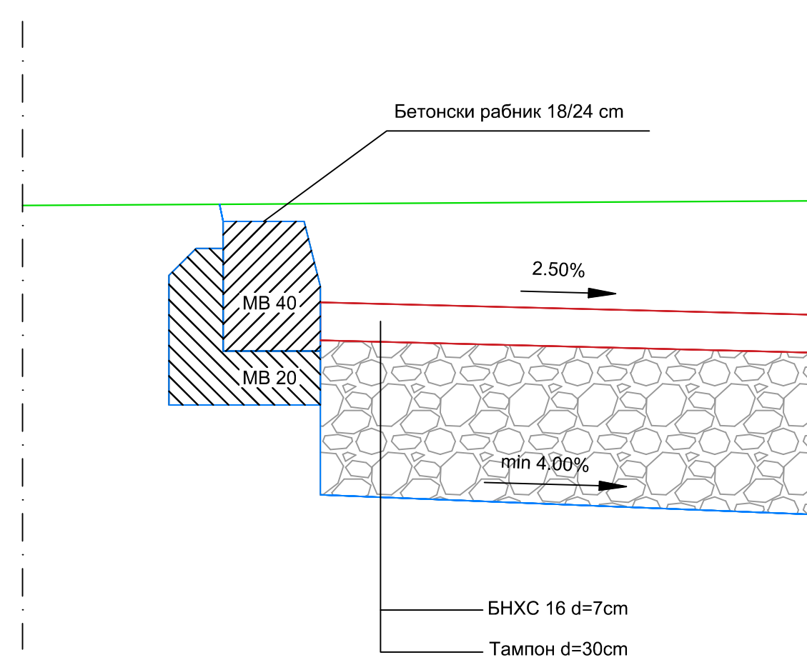
Деталъ "А1" R = 1:10
