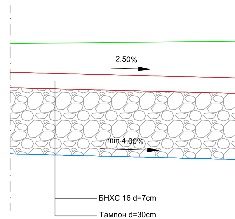
Деталъ "В" - Коловозна конструкција R = 1:10
