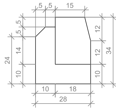
Деталъ за рабник со димензии 18/24/100 cm R = 1:10
