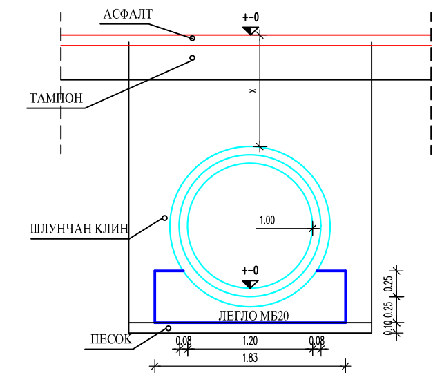
ПРЕСЕК M=1:50
