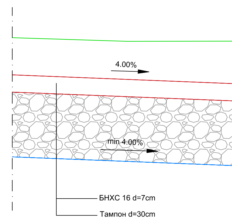
Деталъ "В1" - Коловозна конструкција R = 1:10
